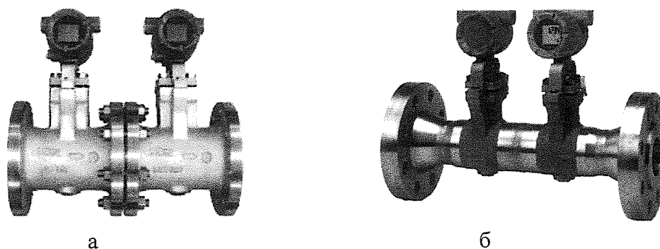
Фото 2 - Фотография общего вида расходомера с двойным сенсором. (а – болтовое соединение, б – сварное соединение)
